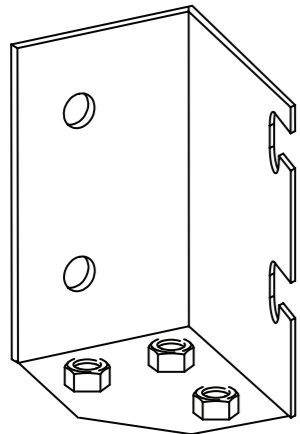
2x BLACHA ŁÓŻKA W-180-105-Z01
