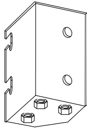
2x BLACHA ŁÓŻKA W-180-105-Z02
